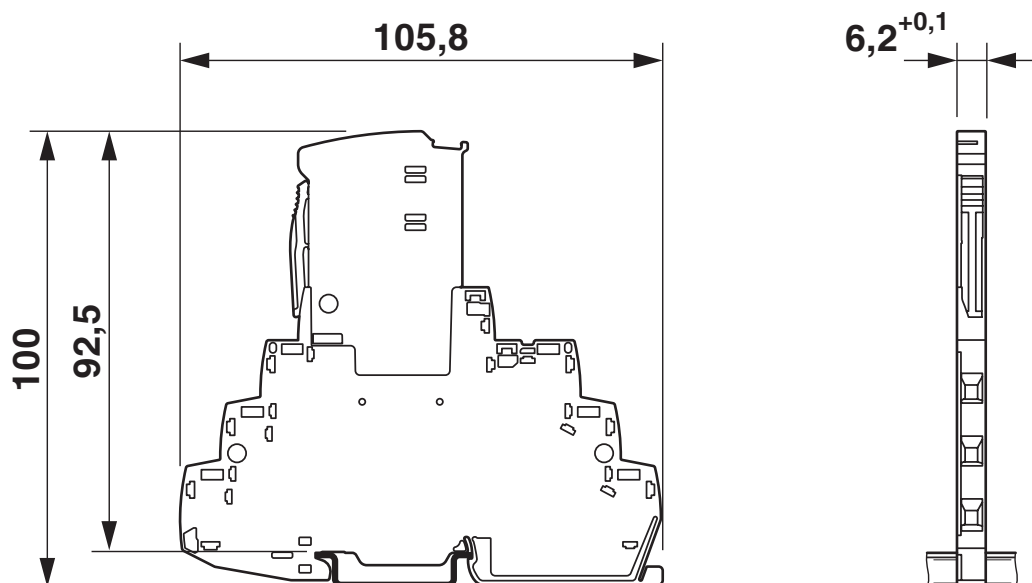
Rysunek wymiarowy
