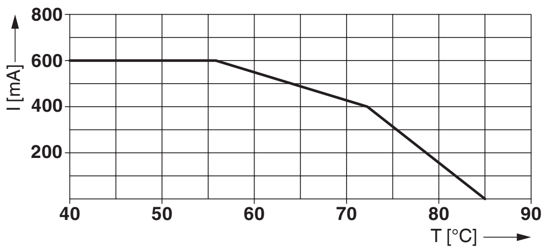
Wykres obniżenia parametrów znamionowych przy 30 V AC
