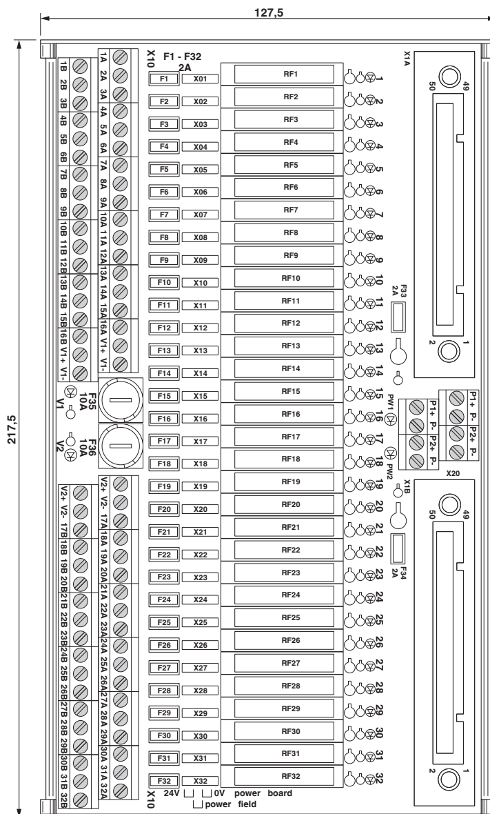
Rysunek wymiarowy
