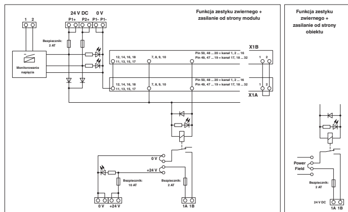
Schemat
