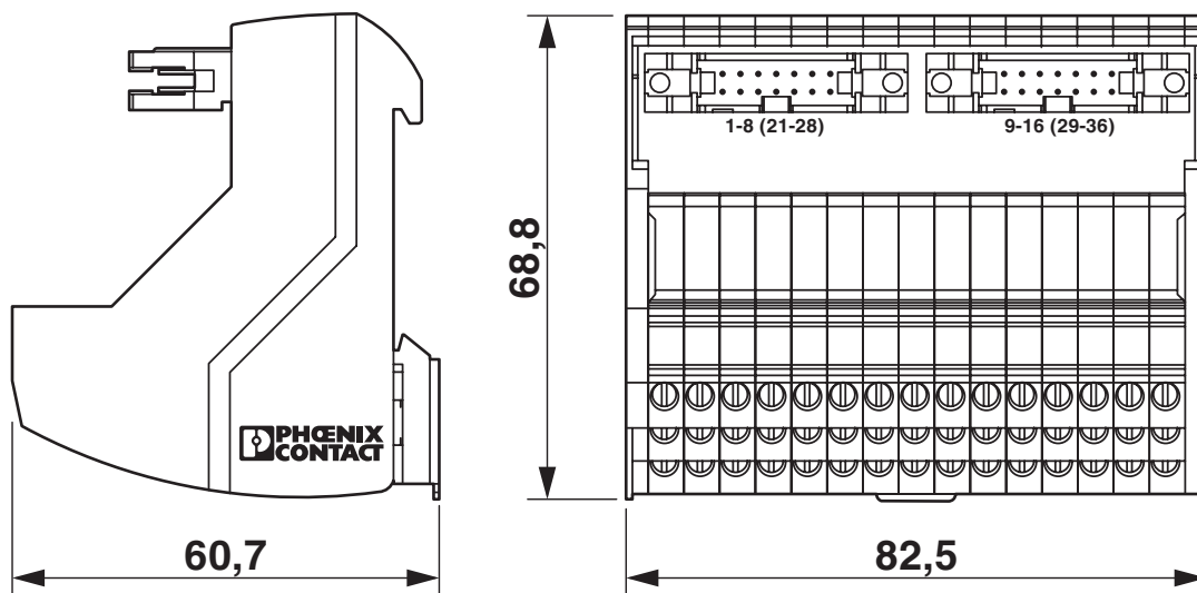
Rysunek wymiarowy
