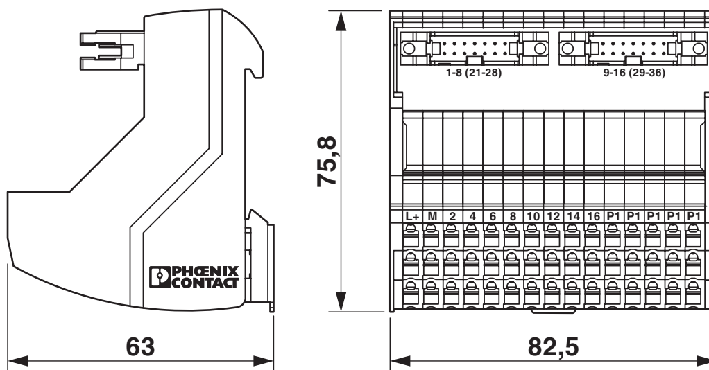
Rysunek wymiarowy
