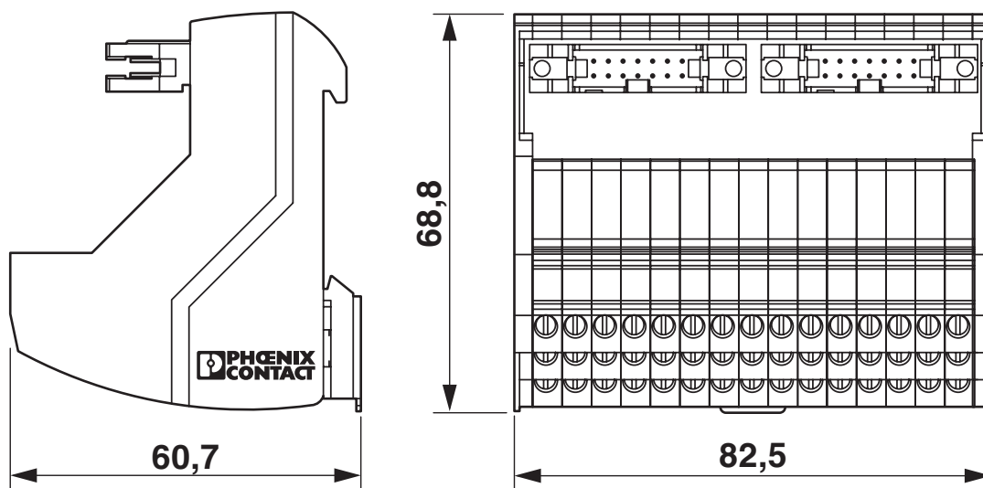
Rysunek wymiarowy
