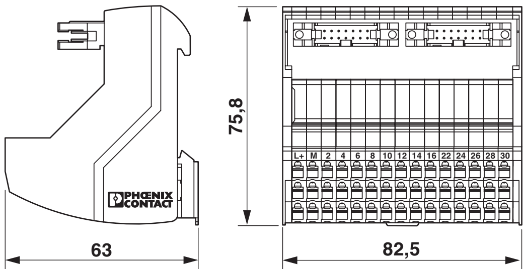
Rysunek wymiarowy
