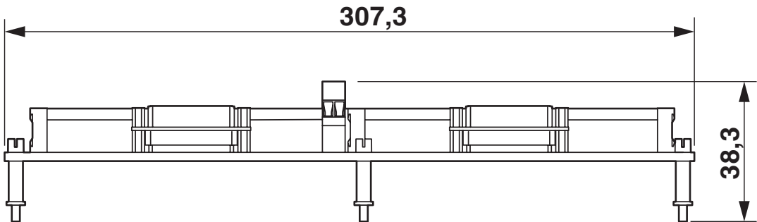
Rysunek wymiarowy
