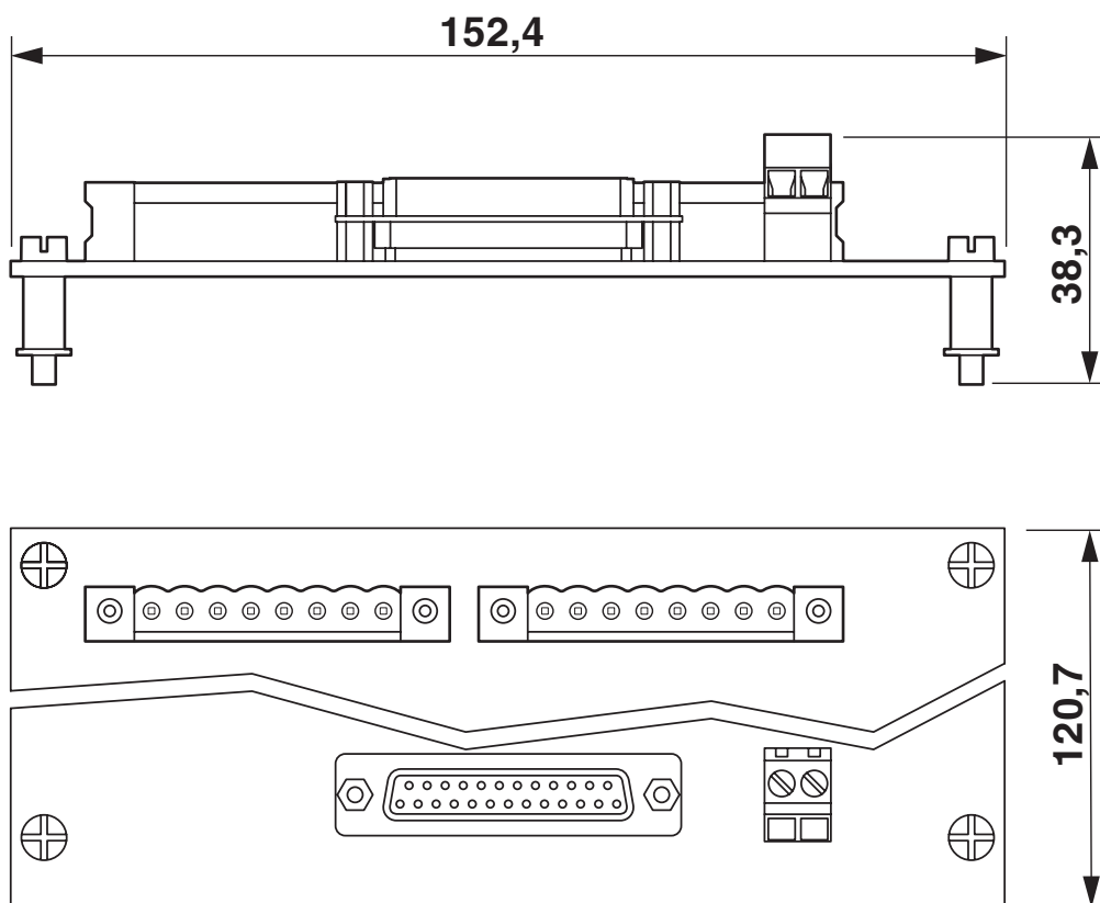
Rysunek wymiarowy
