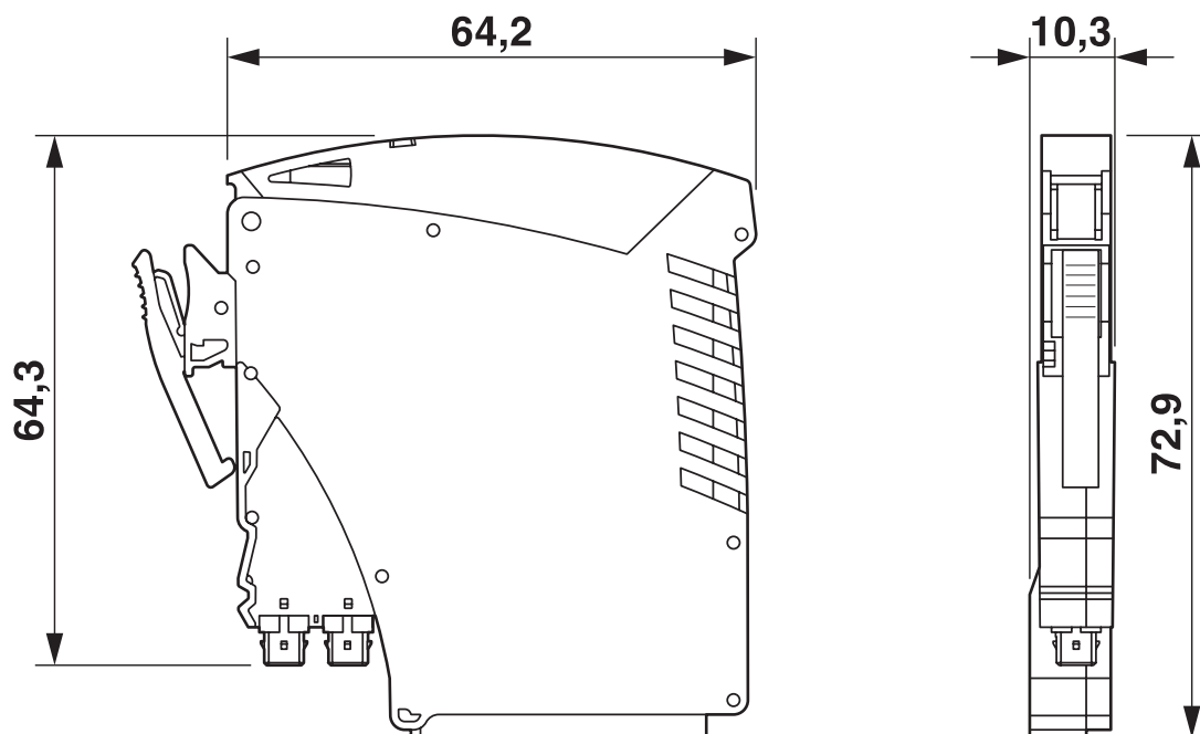
Rysunek wymiarowy
