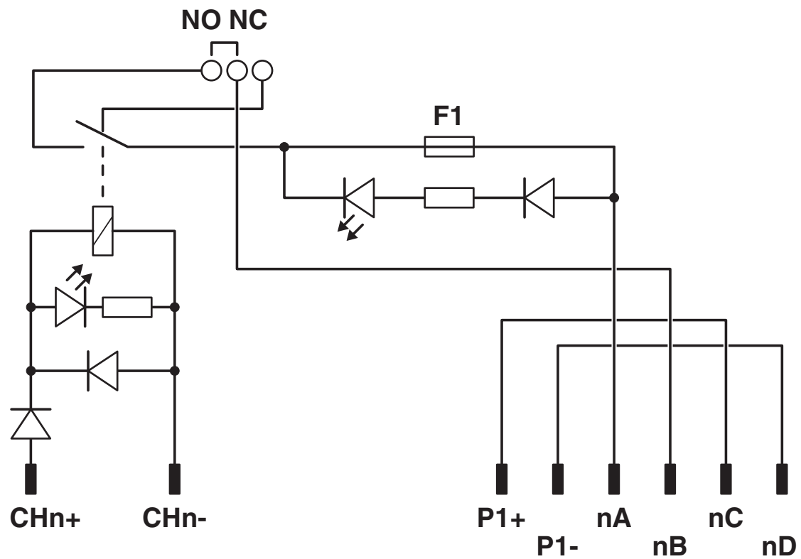
Schemat
