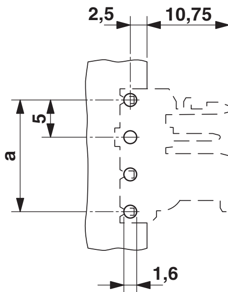
Otworowanie/geometria płytek lutowniczych
