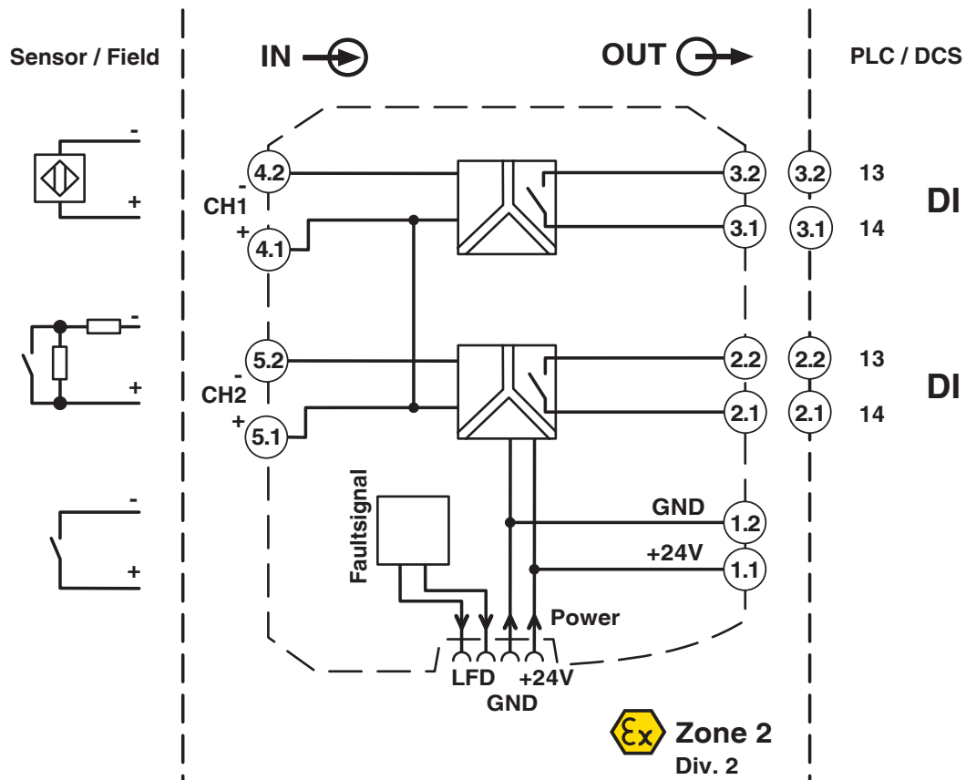
Schemat blokowy
