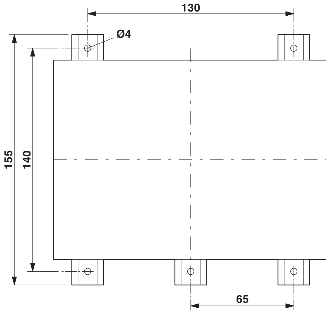
Rysunek wymiarowy
