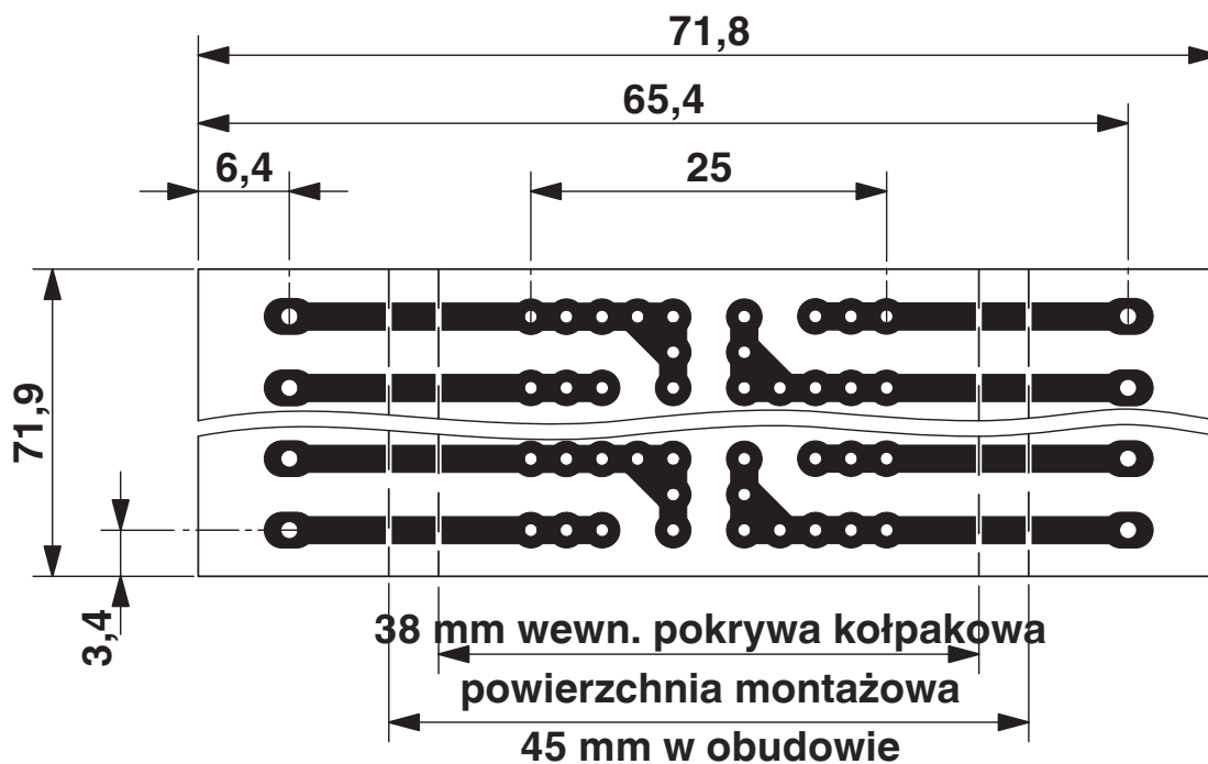
Rysunek wymiarowy
