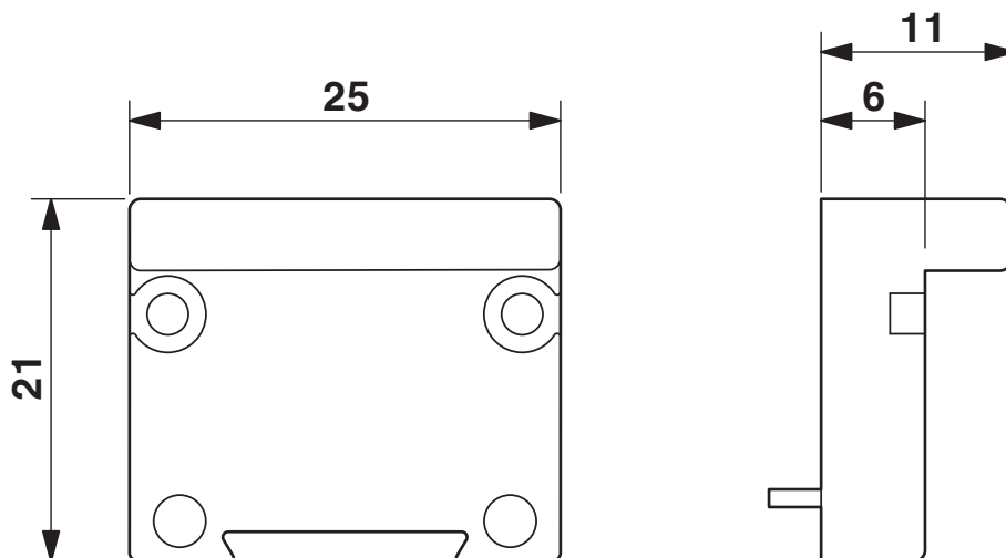
Rysunek wymiarowy
