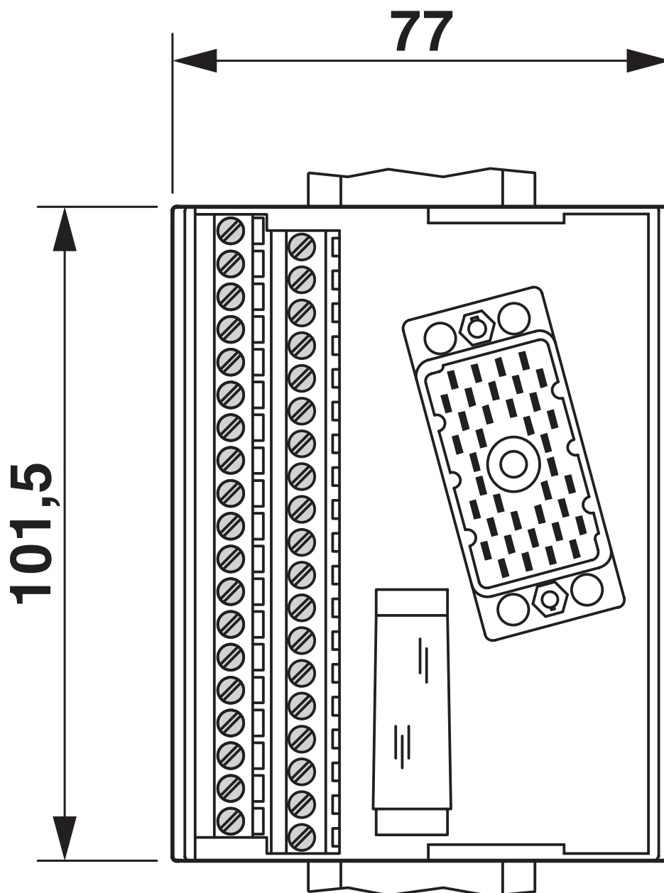
Rysunek wymiarowy
