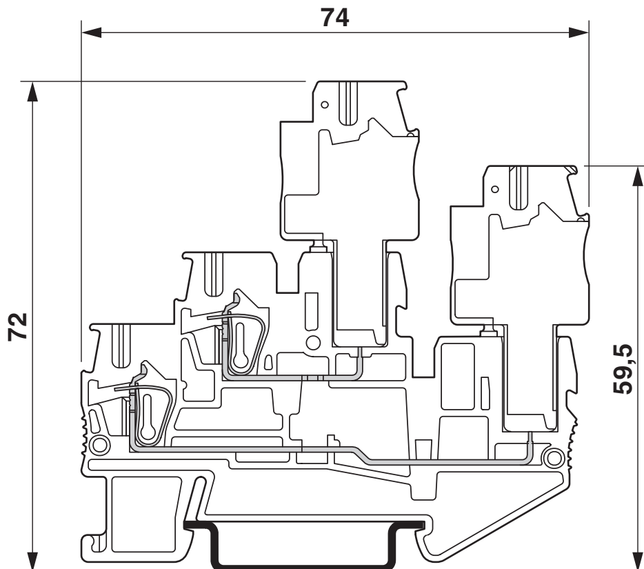
Rysunek wymiarowy
