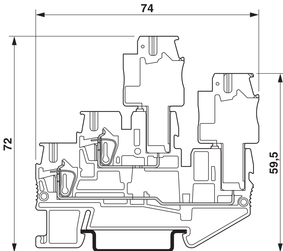
Rysunek wymiarowy
