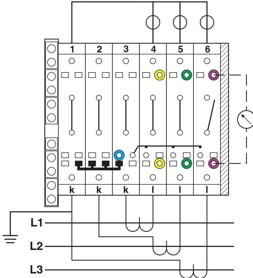
rysunek złączy
