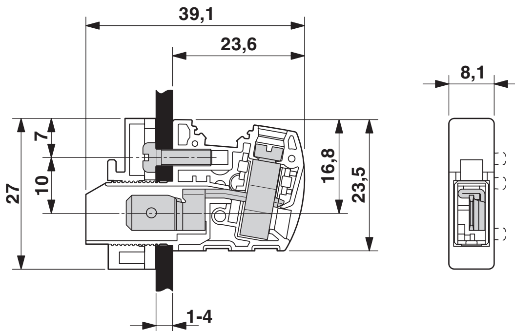
Rysunek wymiarowy
