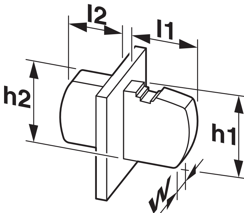
Rysunek wymiarowy
