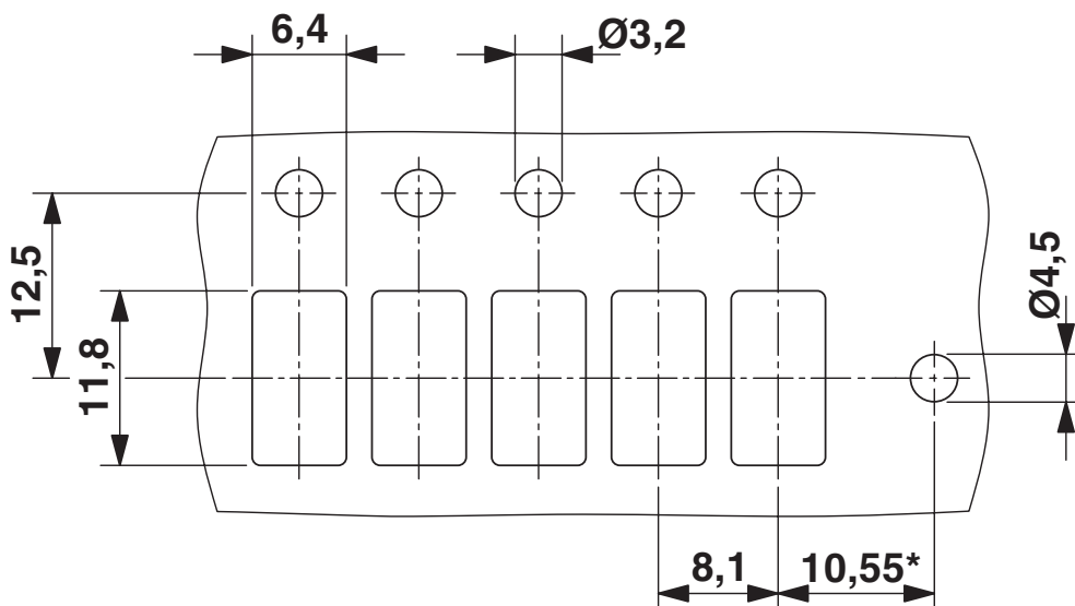
Rysunek wymiarowy
