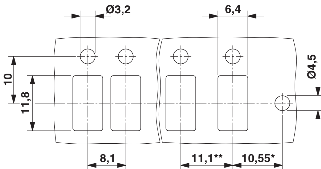
Rysunek wymiarowy
