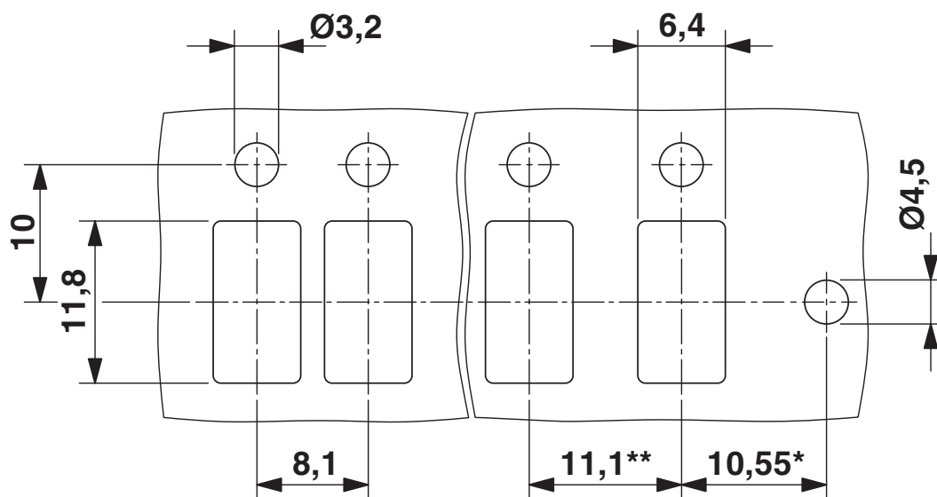
Rysunek wymiarowy
