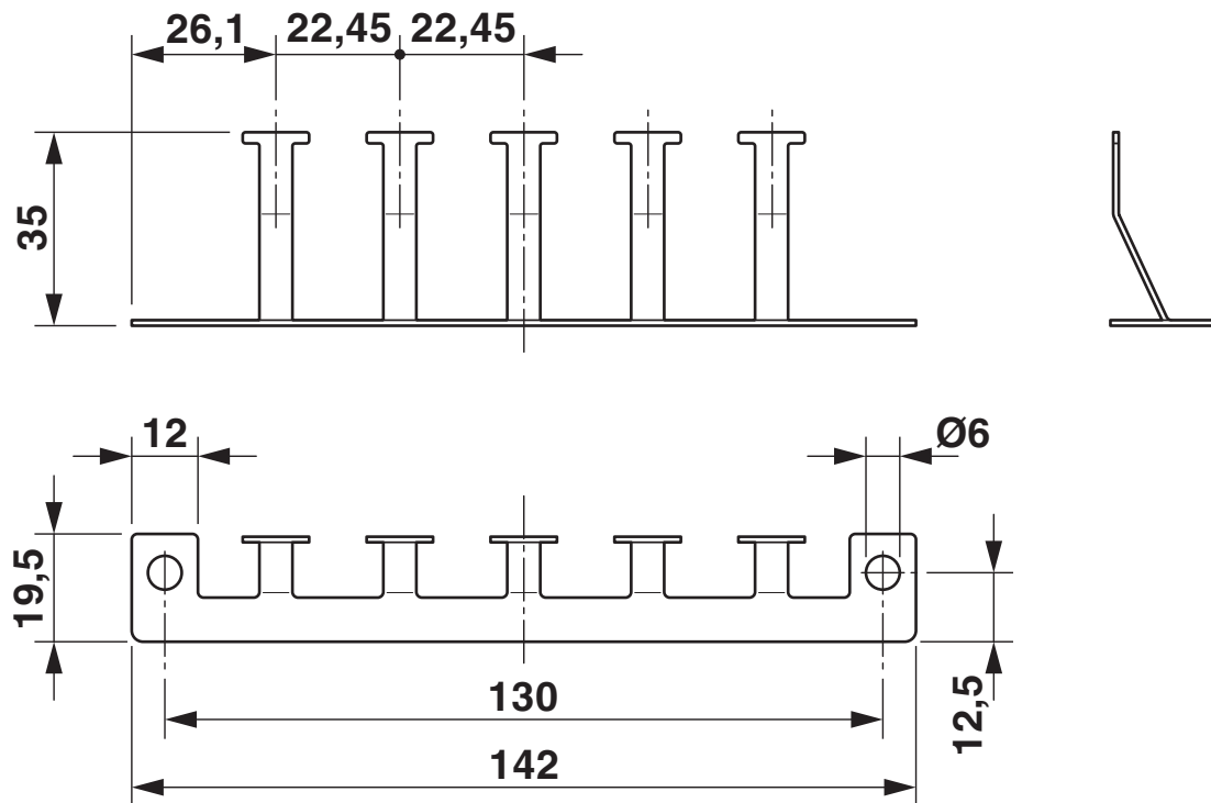
Rysunek wymiarowy
