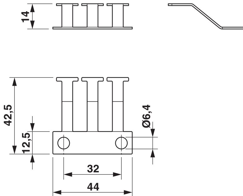
Rysunek wymiarowy
