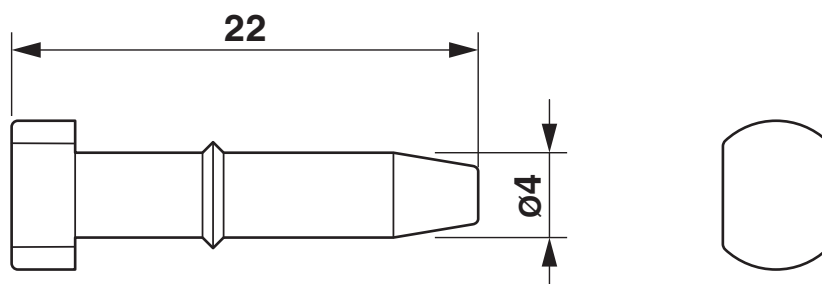
Rysunek wymiarowy
