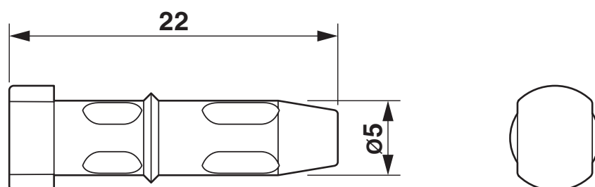
Rysunek wymiarowy
