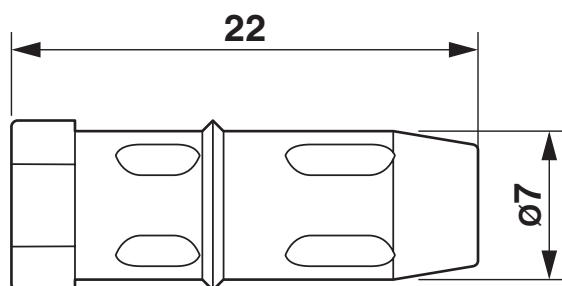
Rysunek wymiarowy
