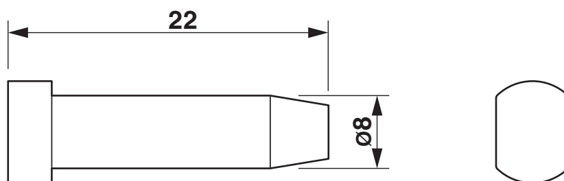
Rysunek wymiarowy
