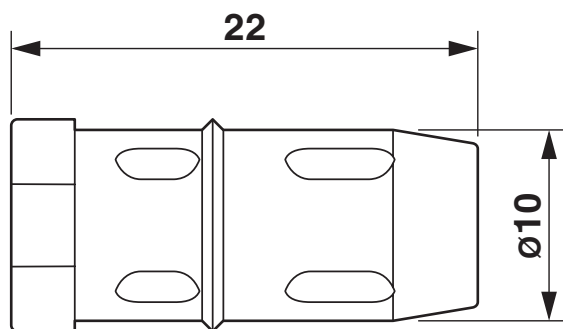
Rysunek wymiarowy
