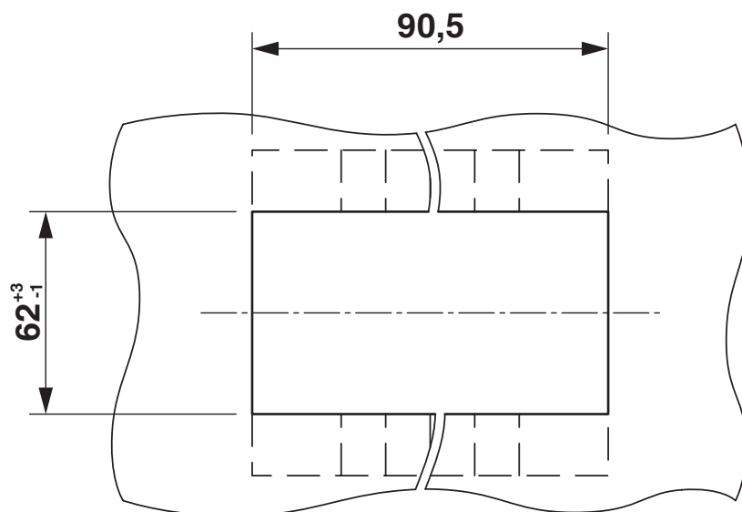
Rysunek wymiarowy
