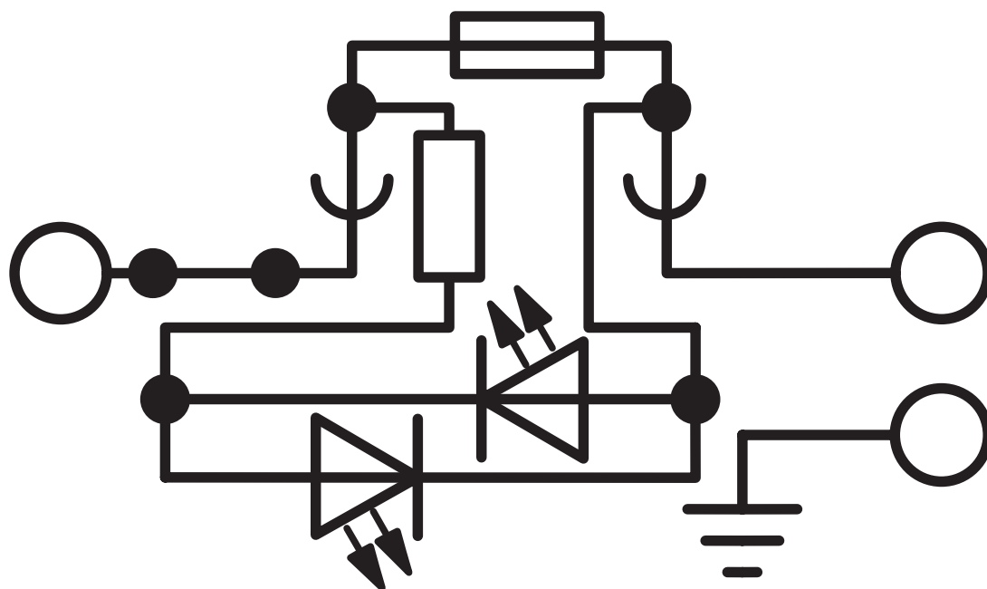
Schemat
