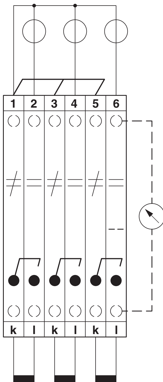
Rysunek schematyczny
