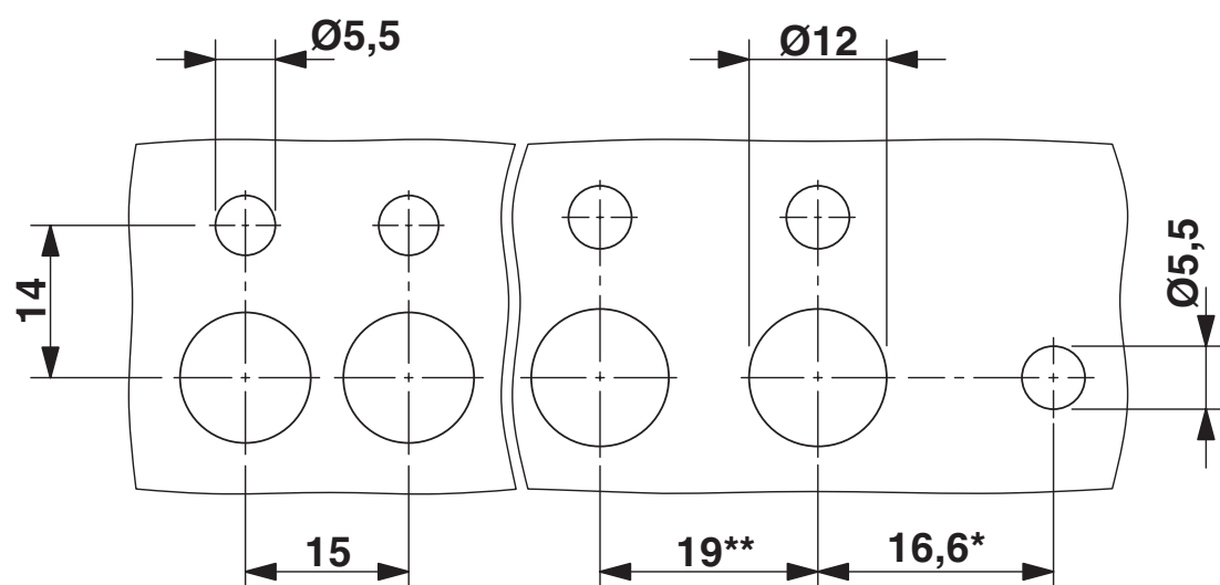
Rysunek wymiarowy
