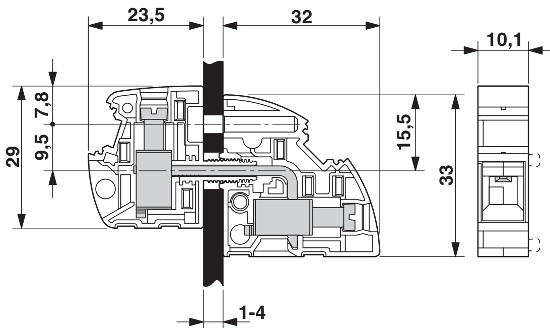
Rysunek wymiarowy
