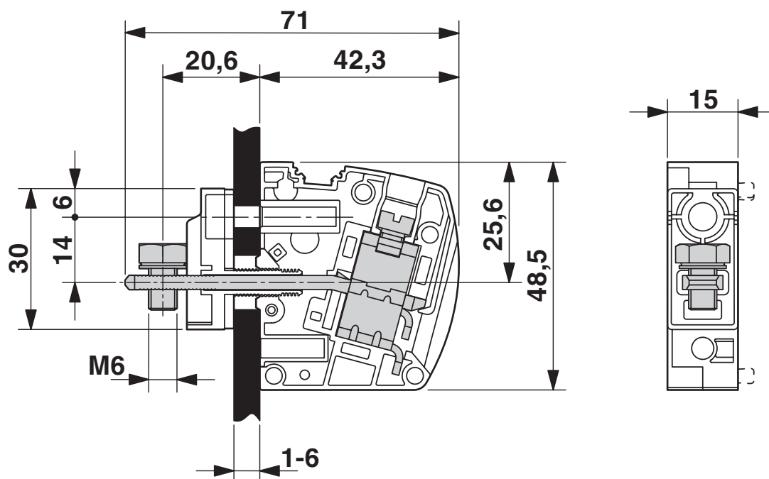
Rysunek wymiarowy
