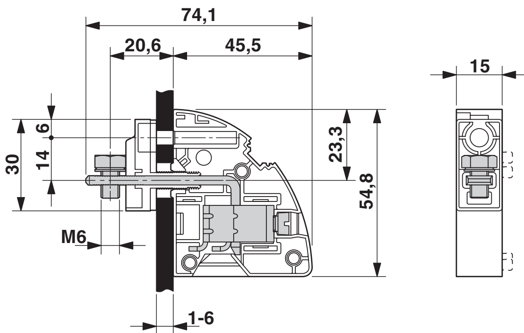
Rysunek wymiarowy
