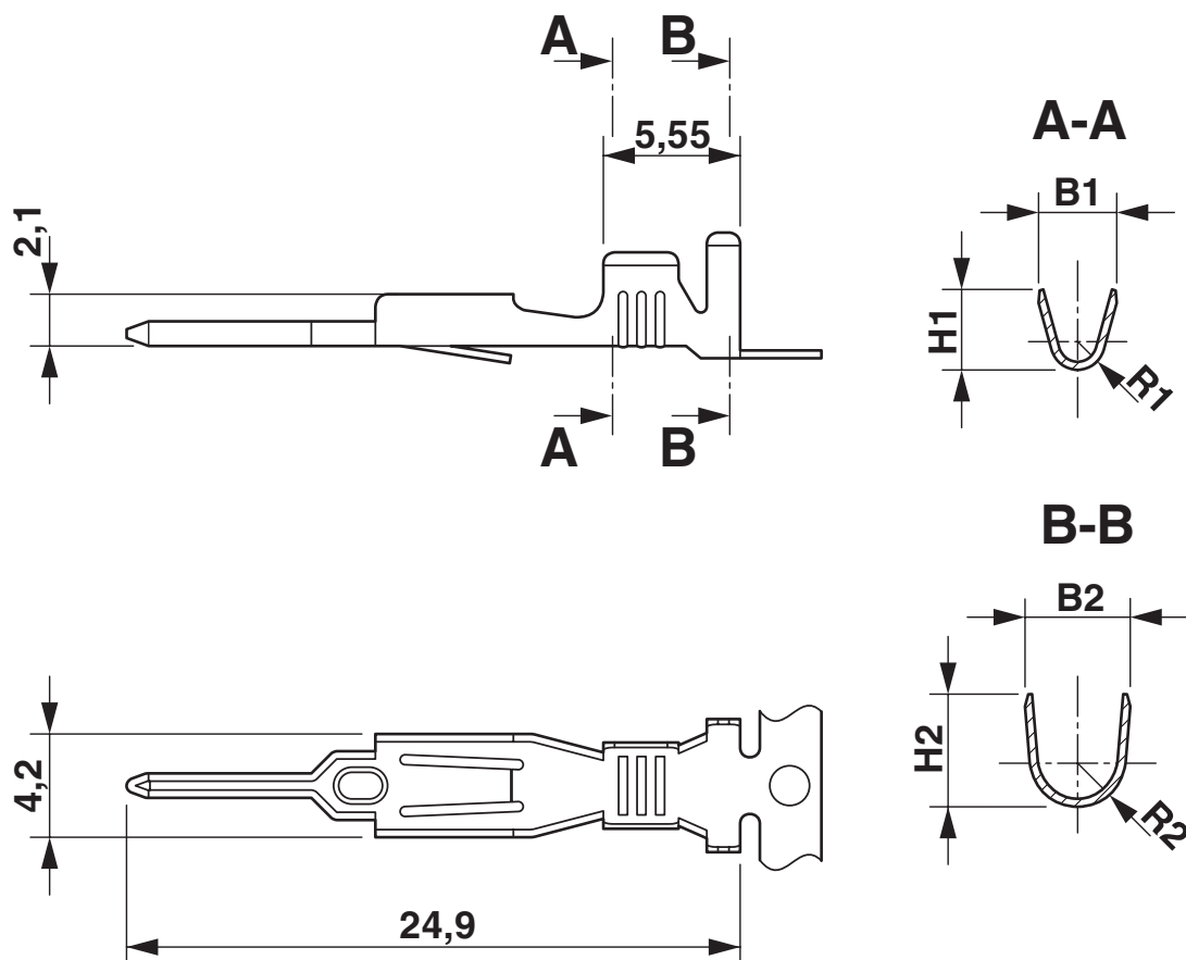
Rysunek wymiarowy
