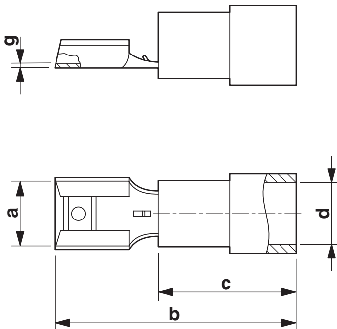
Rysunek wymiarowy
