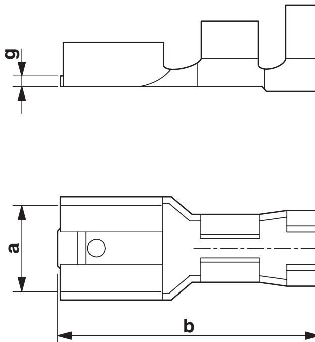
Rysunek wymiarowy
