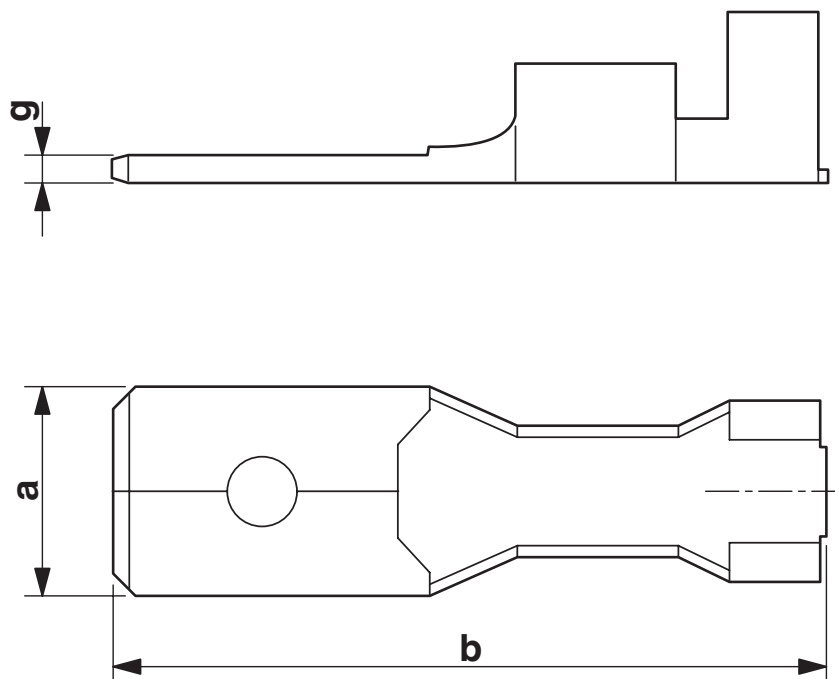
Rysunek wymiarowy
