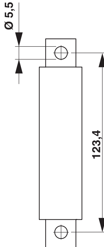
Rysunek wymiarowy
