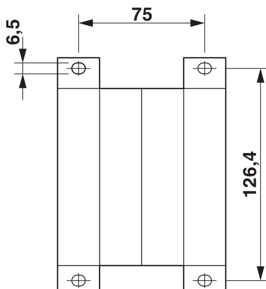
Rysunek wymiarowy
