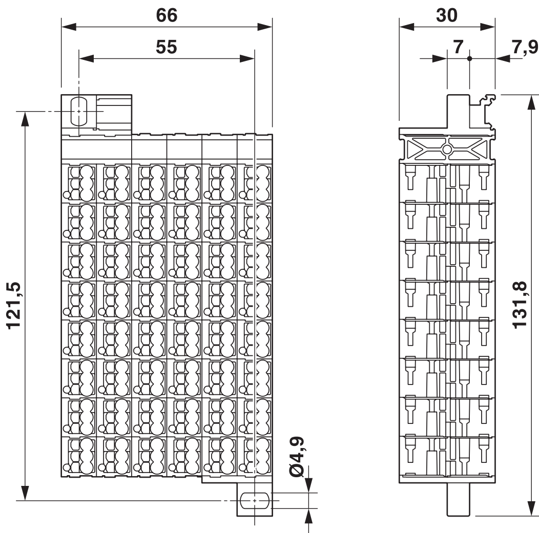
Rysunek wymiarowy
