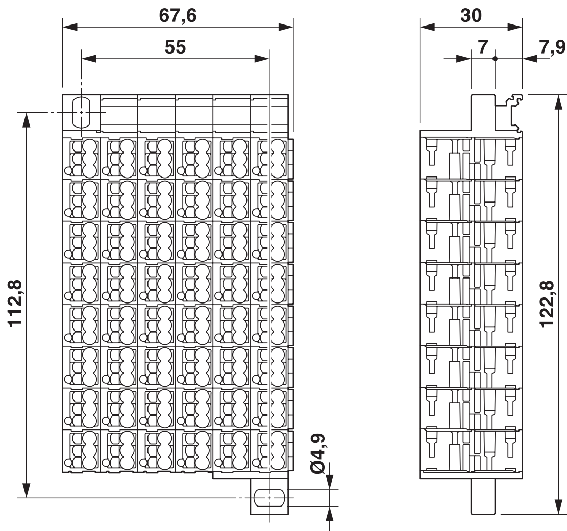
Rysunek wymiarowy
