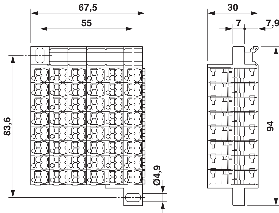
Rysunek wymiarowy
