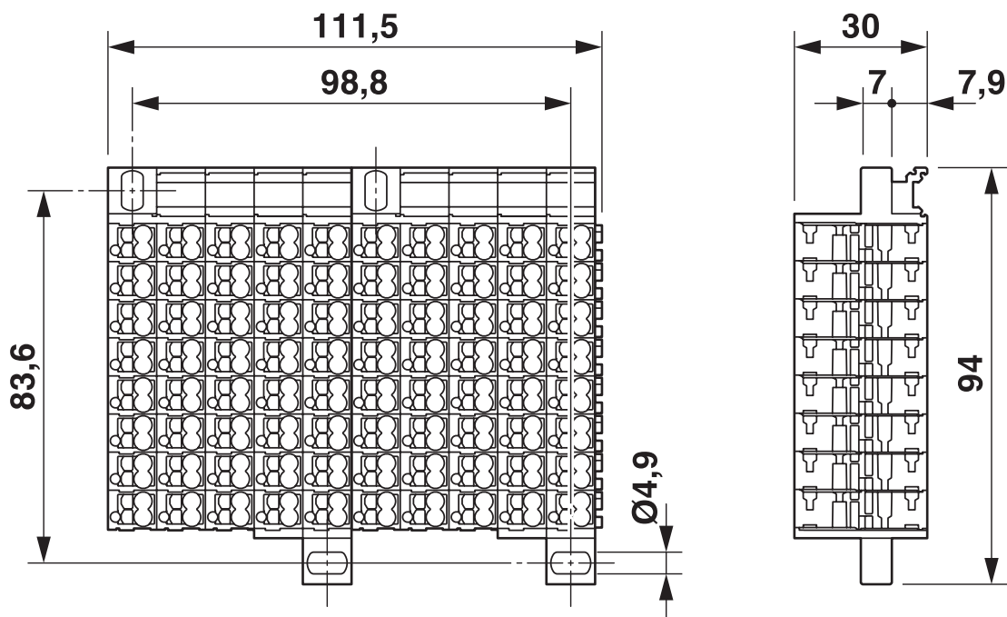
Rysunek wymiarowy
