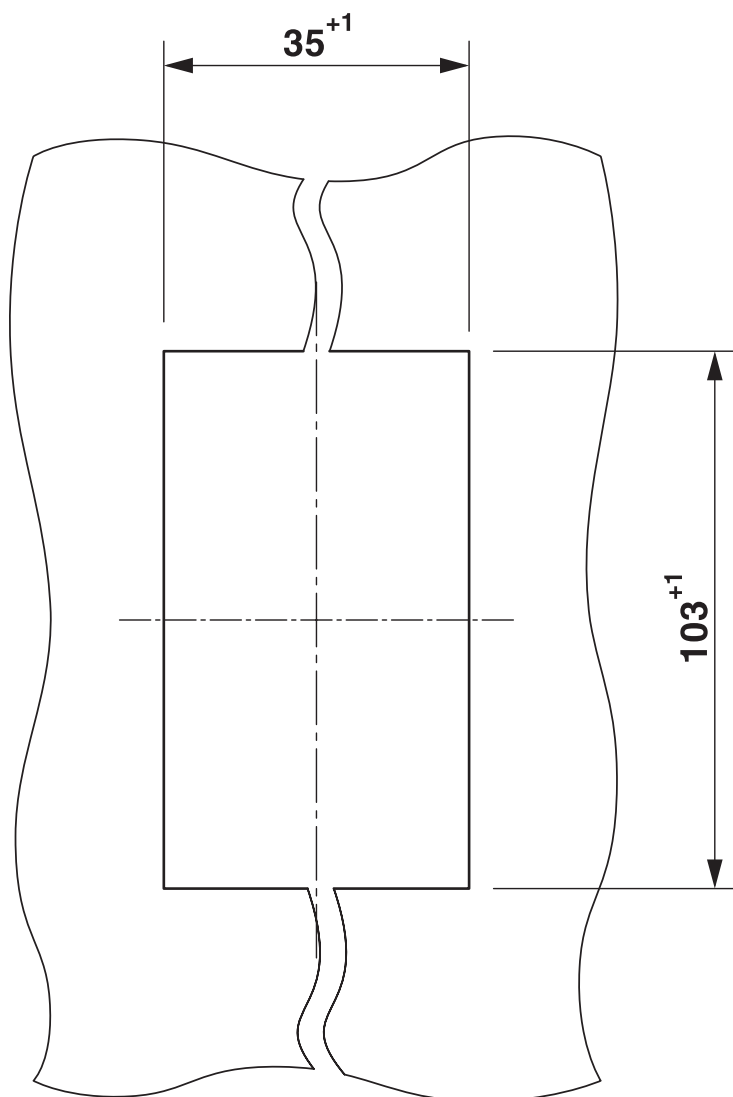
Rysunek wymiarowy
