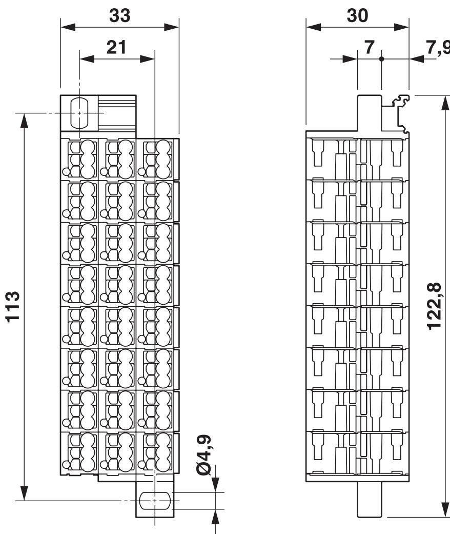
Rysunek wymiarowy
