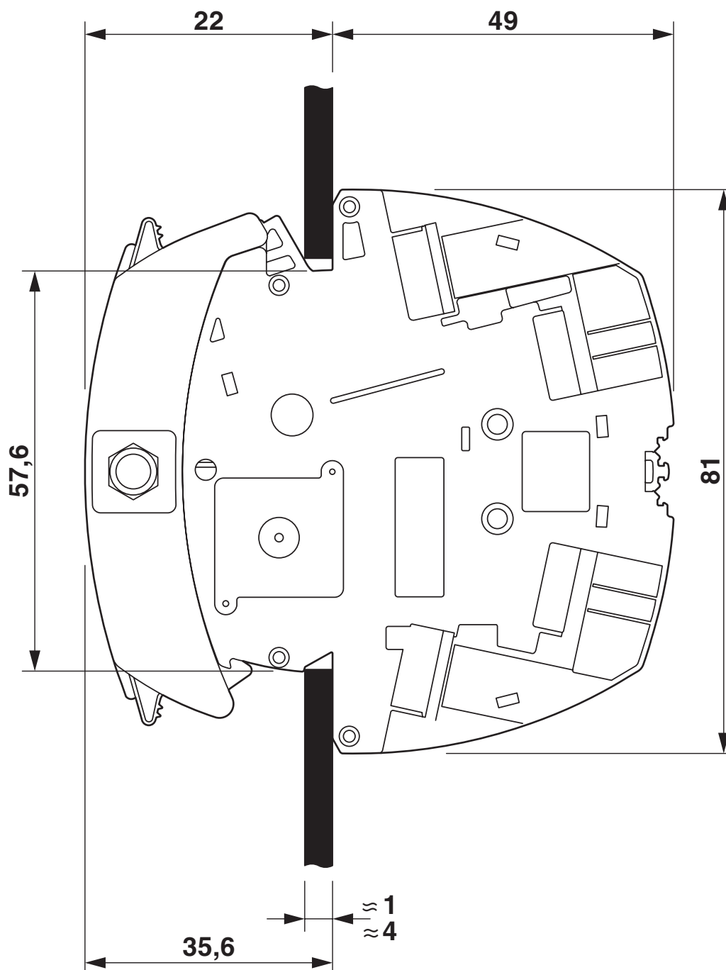
Rysunek wymiarowy
