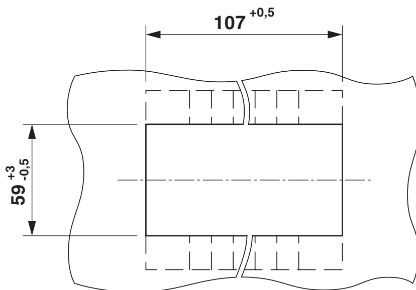
Rysunek wymiarowy
